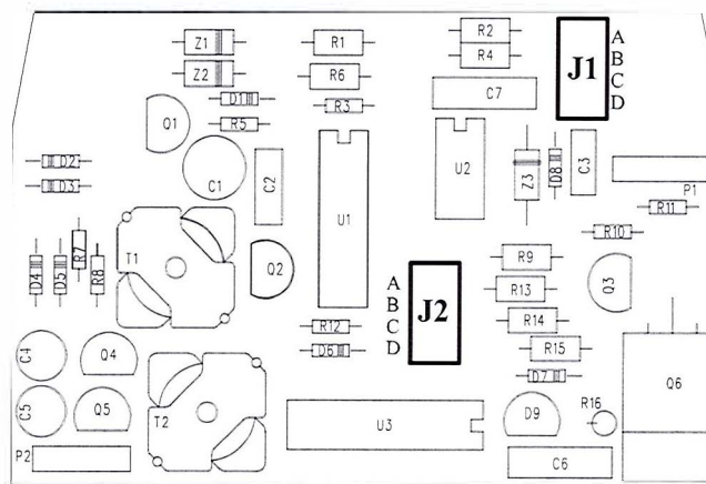
Output PCB
