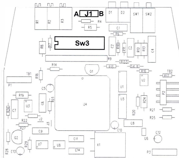
Input PCB
